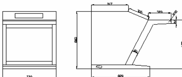
图 4.4-1 SP071 立式操作台示意图
