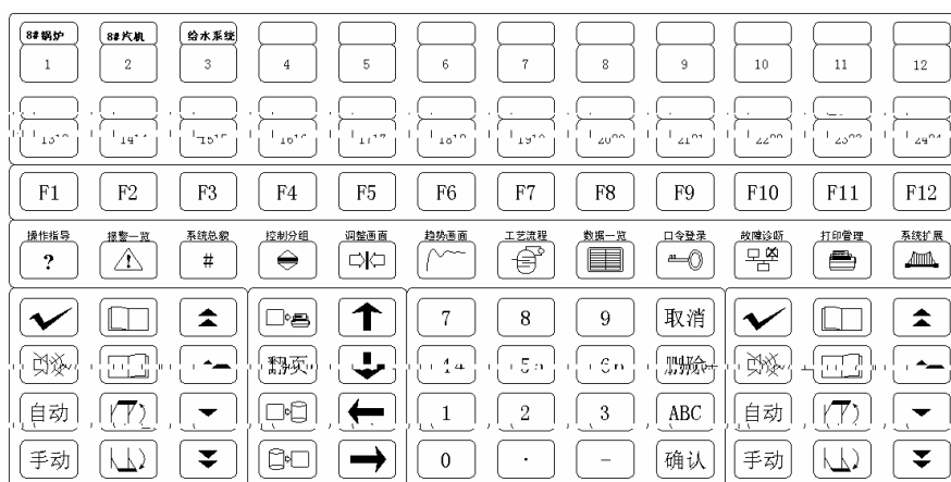
图 4.2-1 操作员键盘
