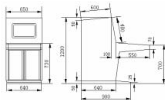
图 4.4-1 SP071 立式操作台示意图
