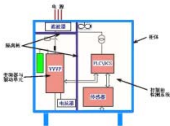
图 1-1 变频控制柜的基本布局
