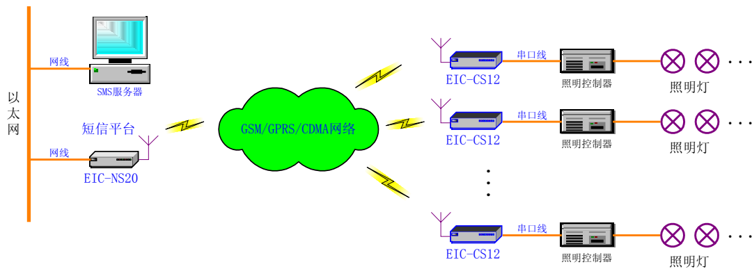
图表 4 市政照明工程
