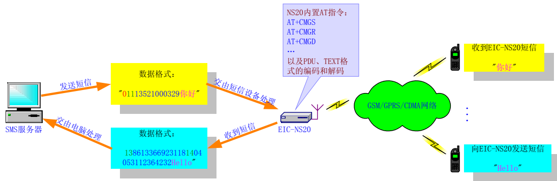
图表 2 NS20 工作原理
