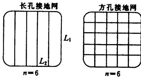
图 B1 接地网的形状
