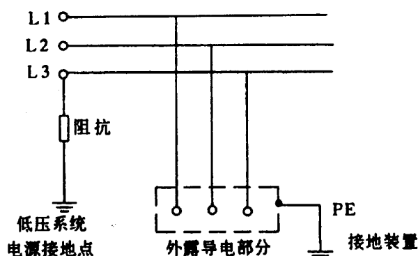
图 5 IT 系统
