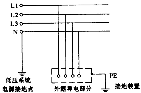
图 4 TT 系统
