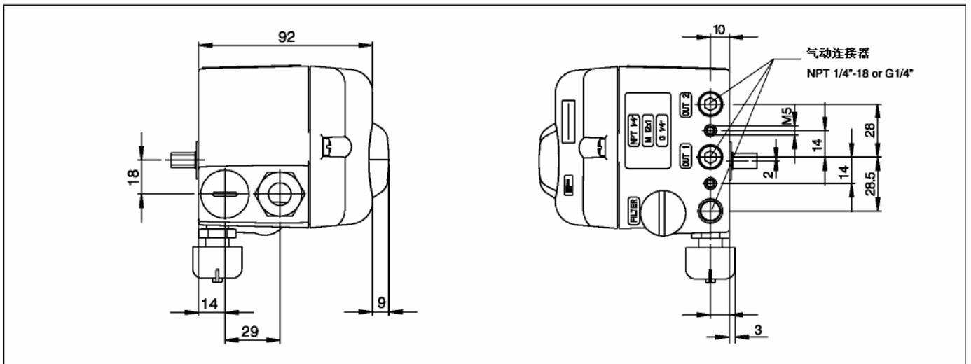
图 14: 左右视图
