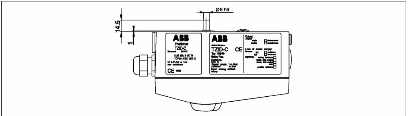
图12: 俯视图
