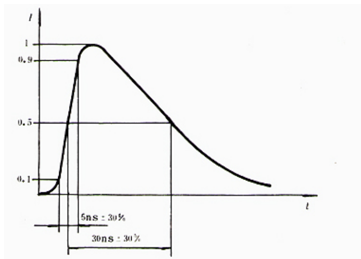
图 7 静电发生器输出电流波形
