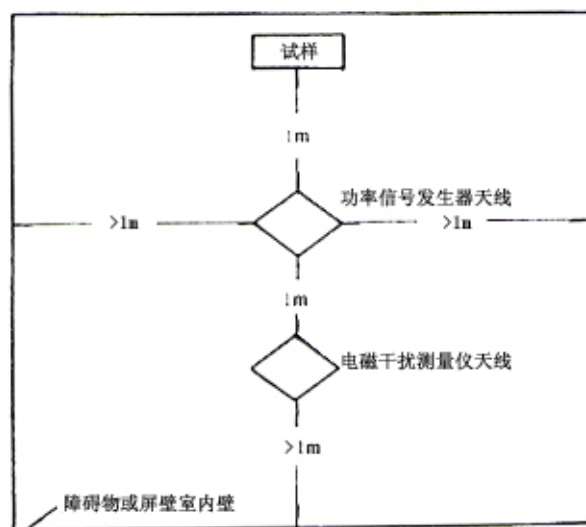
图 9 天线位置图
