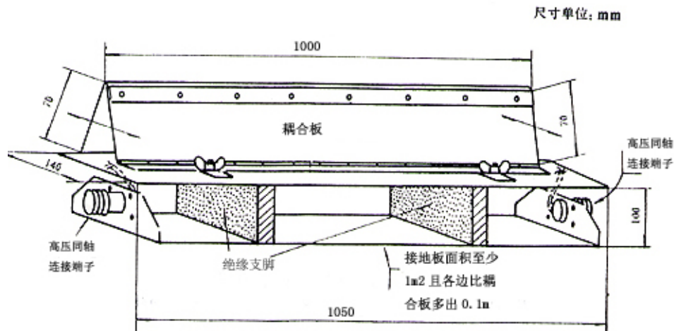
图 5 其他外连接线试验用耦合/去耦网络
