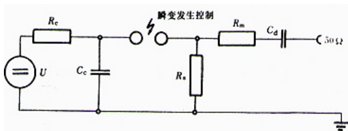
图 3 电瞬变脉冲发生器电原理图
