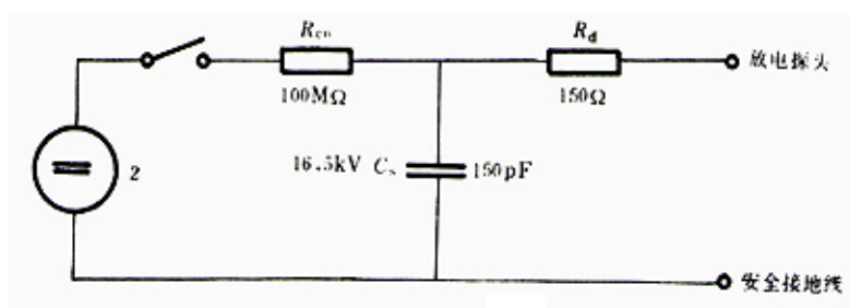
图 6 静电发生器电原理图
