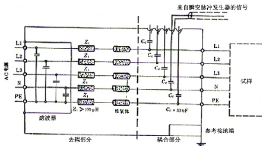
图 4 AC 电源线试验用耦合/去耦网络
