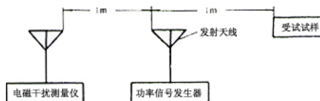
图 8 试验设备布置图
