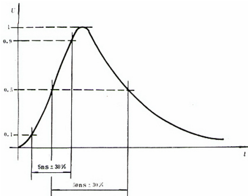
图 1 50Ω 负载时单脉冲波形
